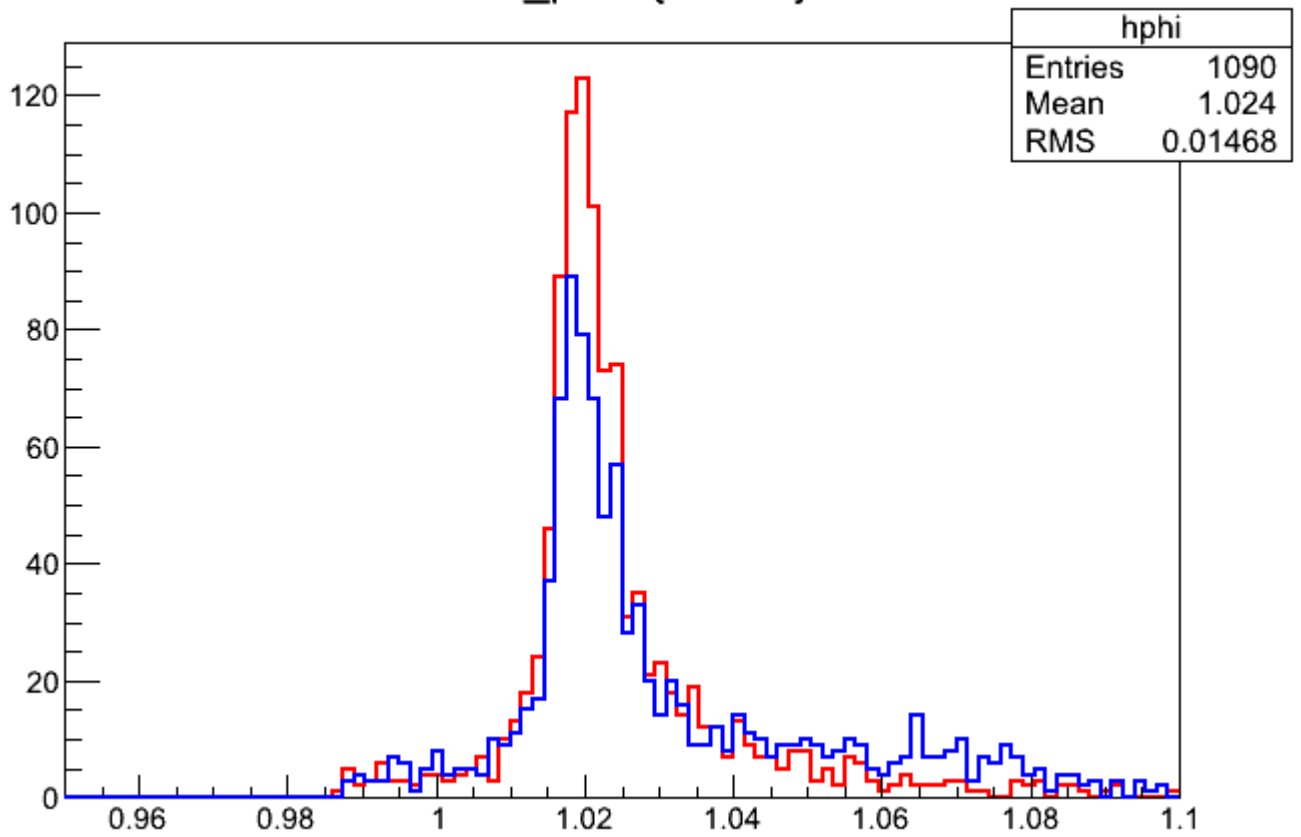
reco_phi1 {eff==4}
