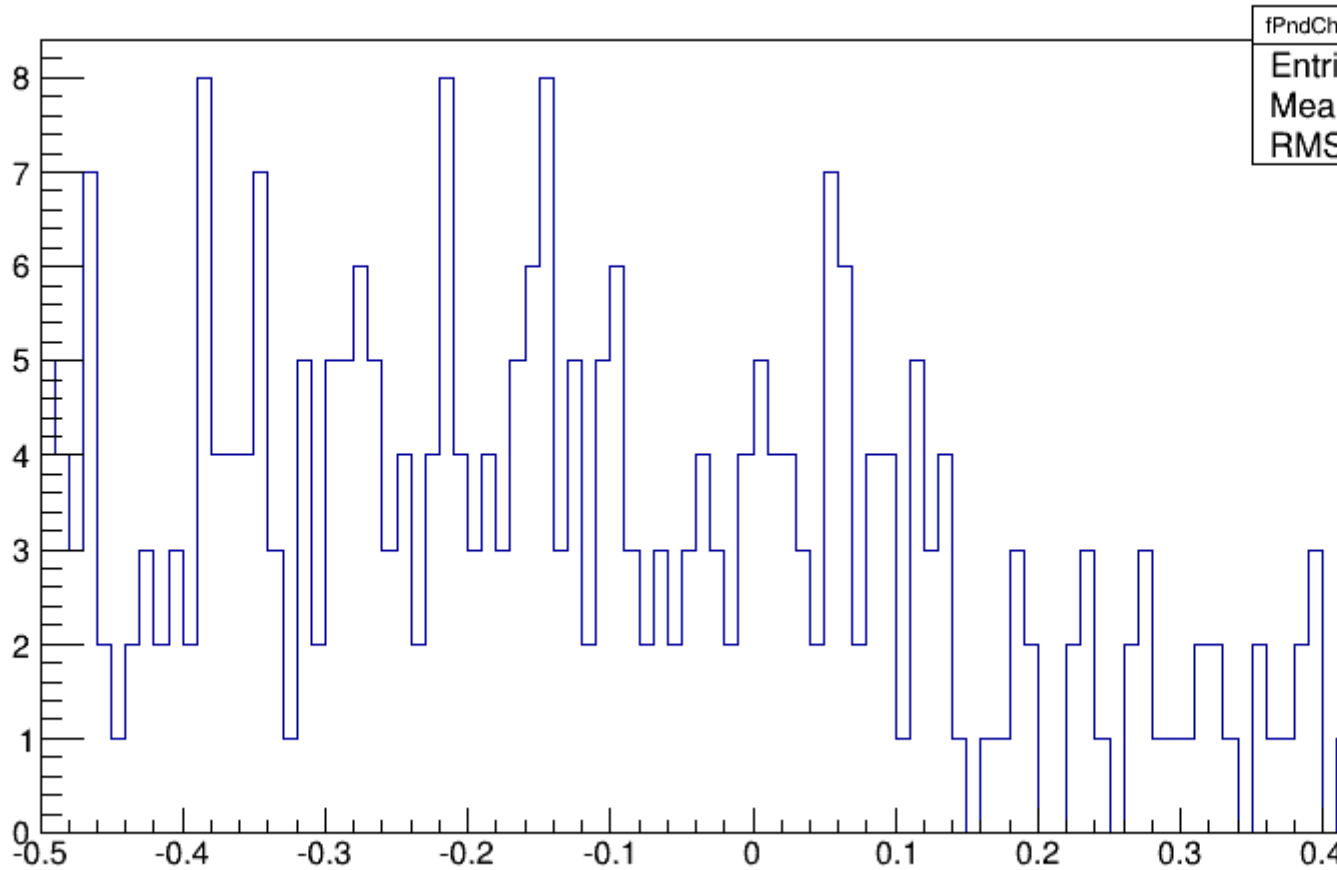
fPndChiVtxFitter_VertexRes_Z
