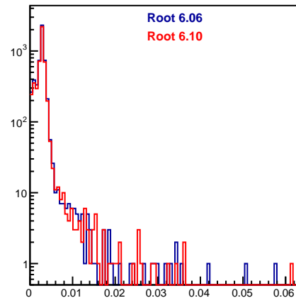
FtofPoint.fELoss
