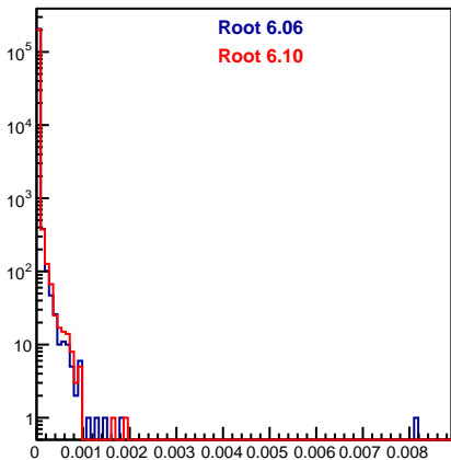
FTSPoint.fELoss
