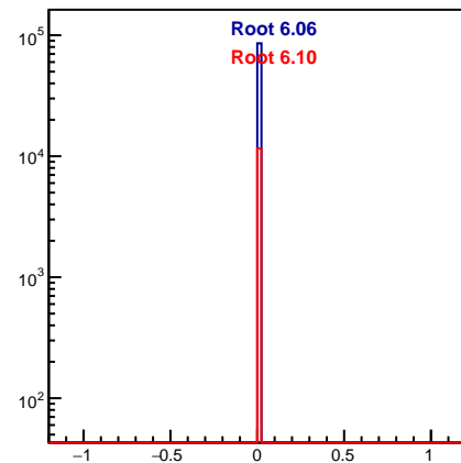
DrcBarPoint.fELoss
