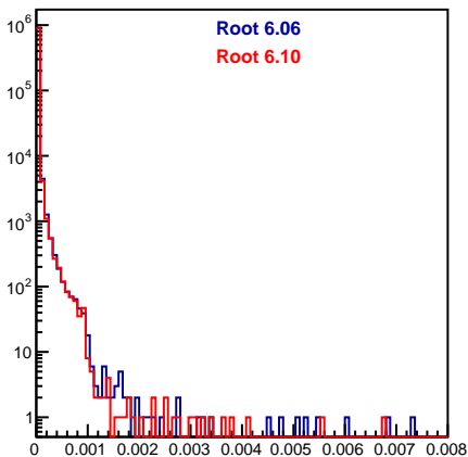
STTPoint.fELoss
