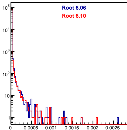
GEMPoint.fELoss
