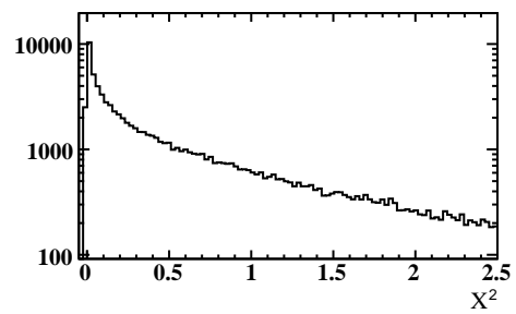
Vertex Kin \chi^2
