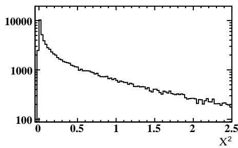
Vertex Fit \chi^2
