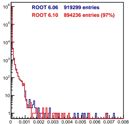
STTPoint.fELoss
