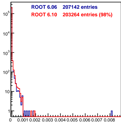
FTSPoint.fELoss
