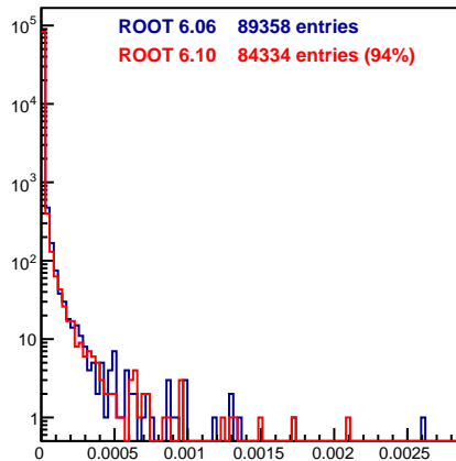
GEMPoint.fELoss
