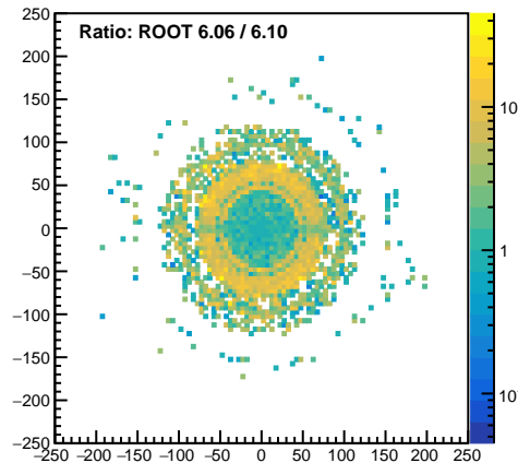
MCTrack.fStartX:MCTrack.fStartY (fStartZ&lt;200)
