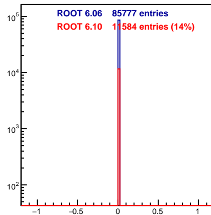
DrcBarPoint.fELoss
