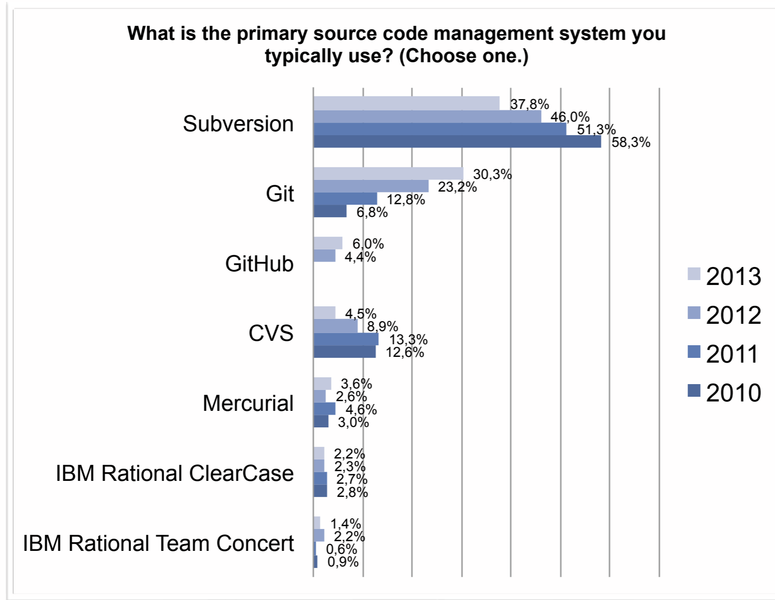
Eclipse IDE survey 2013
