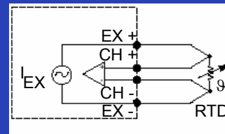
4-Leitungsmessung
