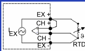
3-Leitungsmessung
