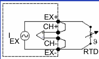
2-Leitungsmessung
